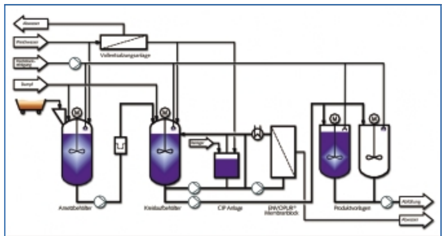
3: Herzstück der Produktion von Flüssigfarbstoffen: die Membrananlage zum Entsalzen und Aufkonzentrieren der Rohlösung
